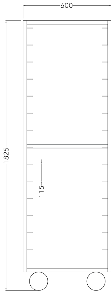
VISTA FRONTAL ESC. 1:12
