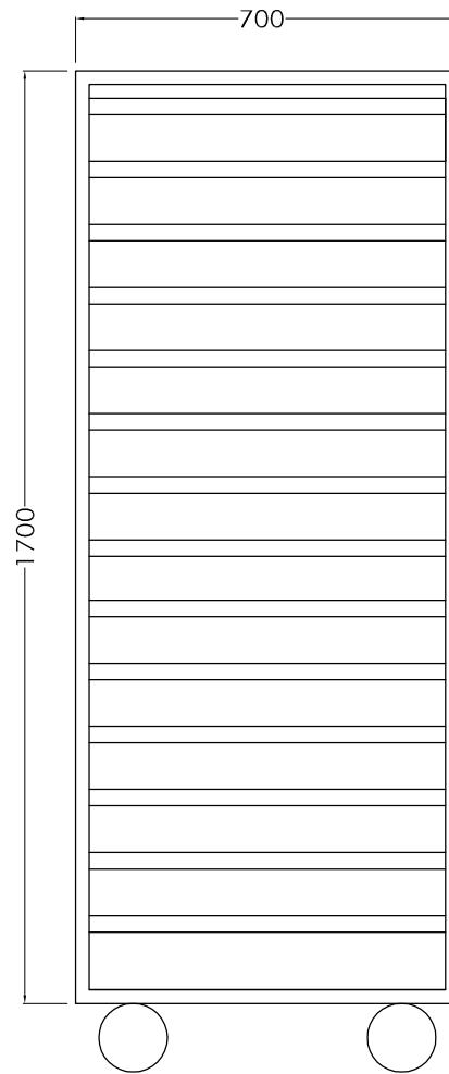
VISTA LATERAL ESC. 1:12
