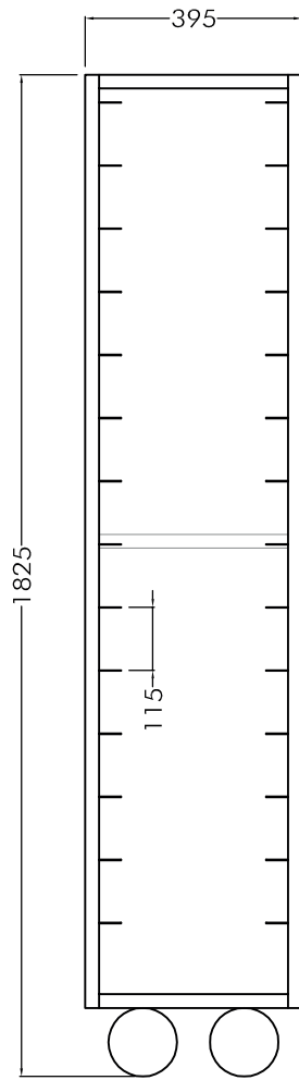
VISTA FRONTAL ESC. 1:12
