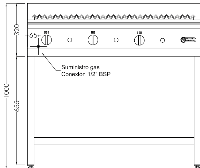
VISTA FRONTAL ESC. 1:15
